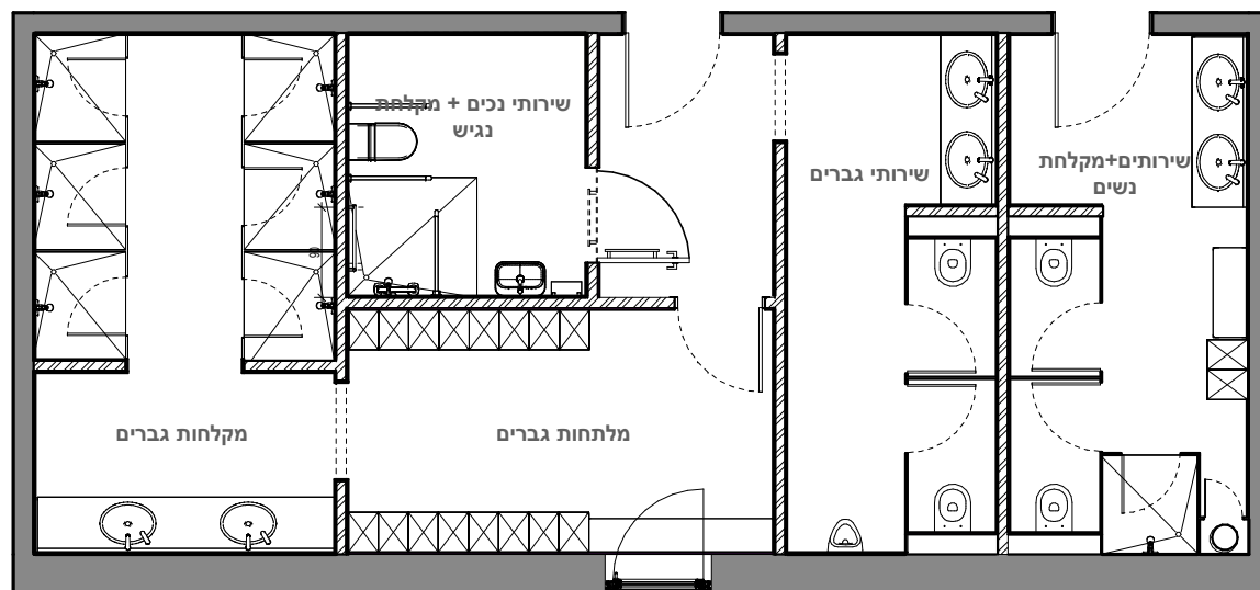
1 תכנית העמדה 1:50
