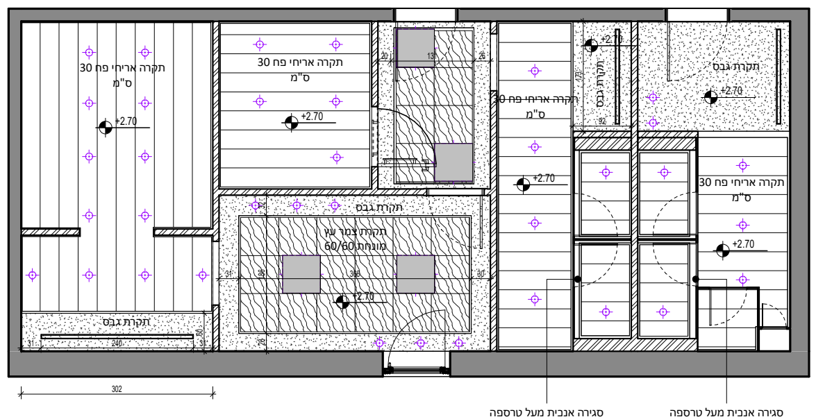
1 תקרה ותאורה 1:50
